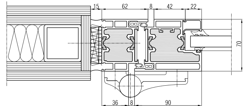
Anschluss an Montagewand
