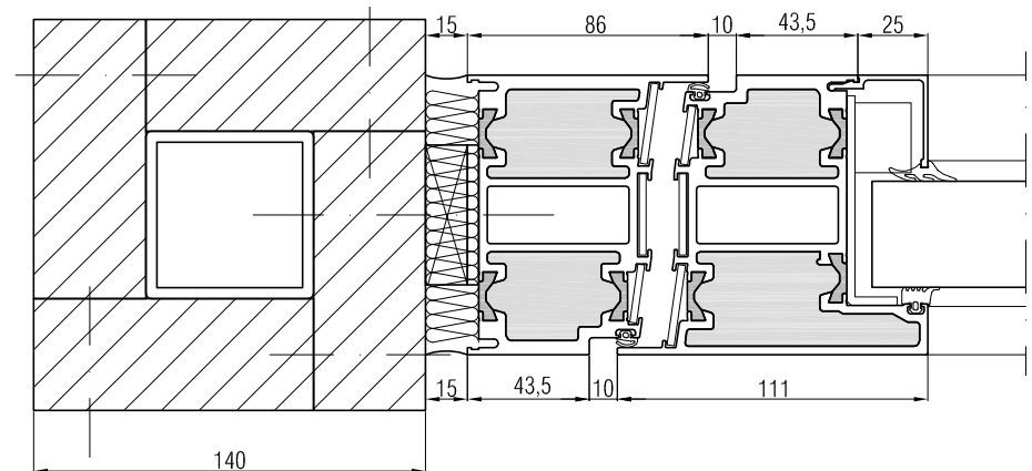
Anschluss an Stütze
