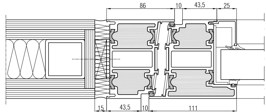
Anschluss an Montagewand
